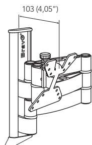
Adattatore 20x10 20x10 Adapter
