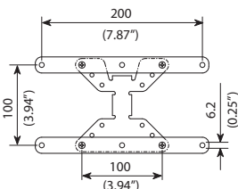
Adattatore 20x10 20x10 Adapter
